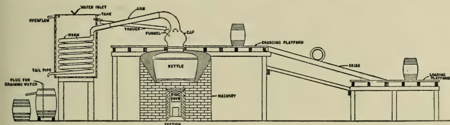
FIG. 79.—Retort for Distilling Rosin.
